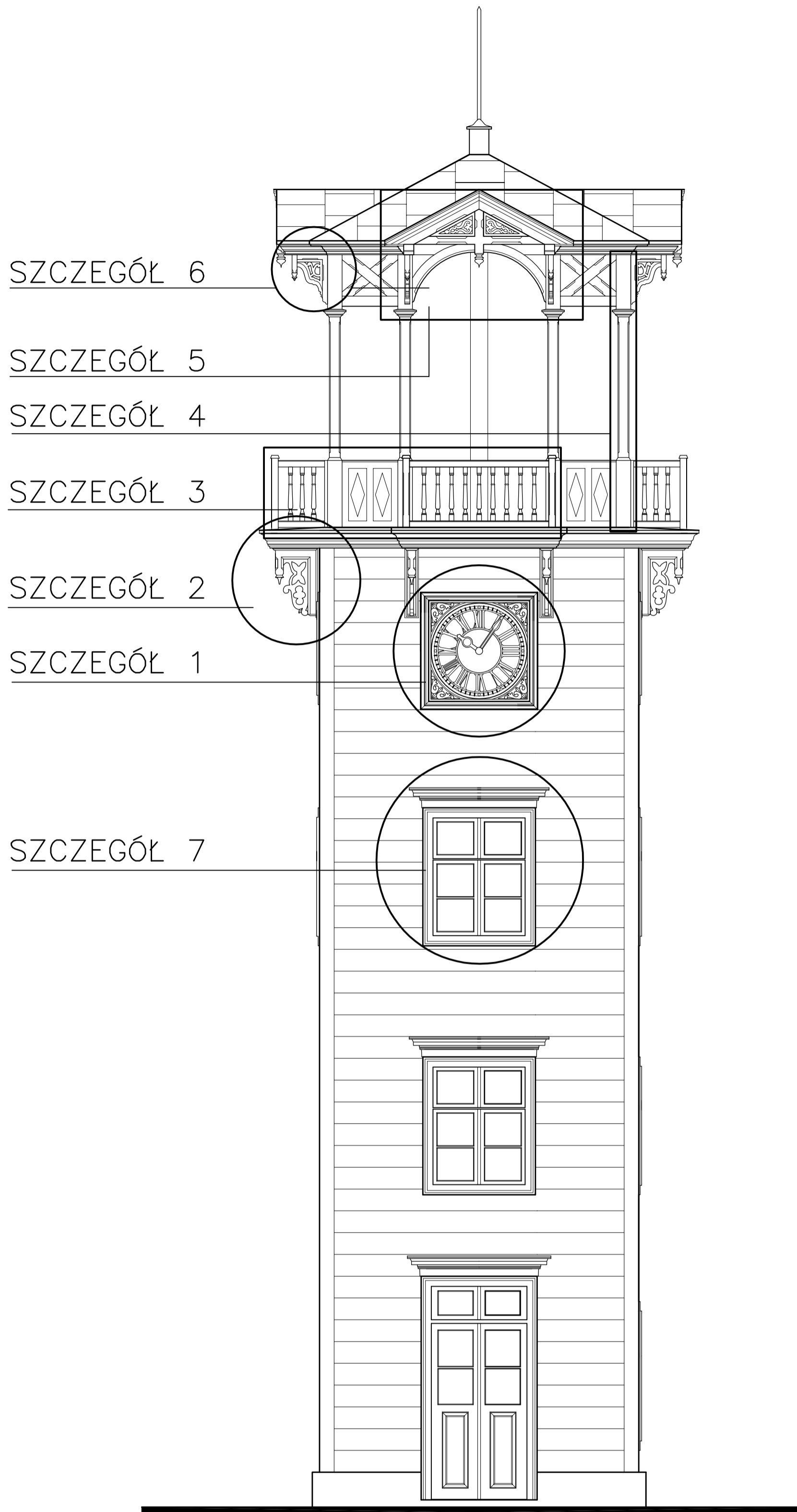
ELEWACJA PÓŁNOCNO – ZACHODNIA
