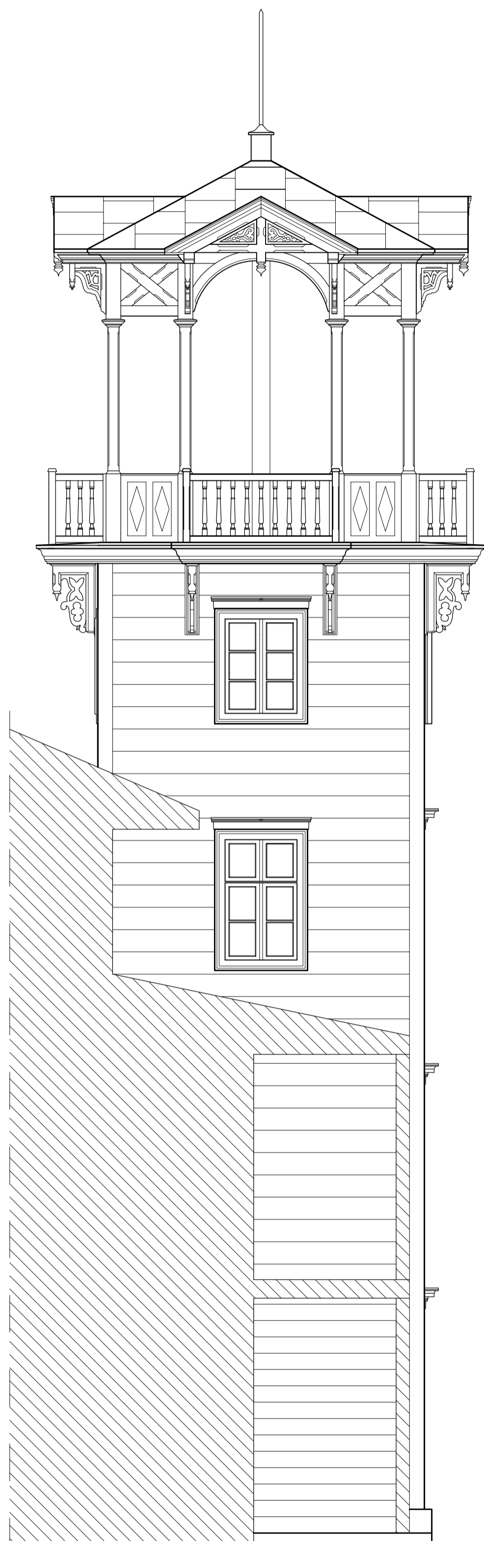
ELEWACJA PÓŁNOCNO – WSCHODNIA
