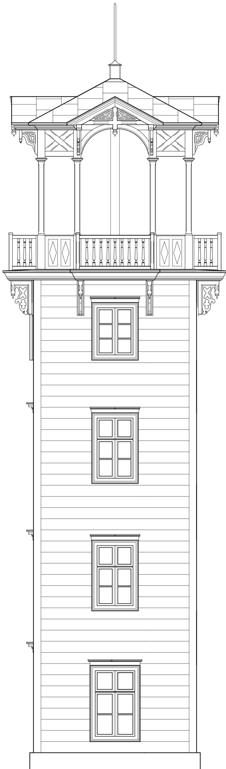
ELEWACJA POŁUDNIOWO – ZACHODNIA
